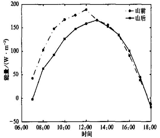
图8 山前山后感热通量日变化图
