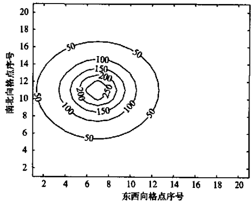
图 1 模式模拟地形高度(单位:m)
