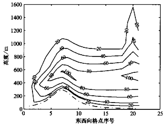
图 5 湍流交换系数的垂直剖面图 (单位: \text{m}^2 \text{ s}^{-1} , 格距为 1 km)
