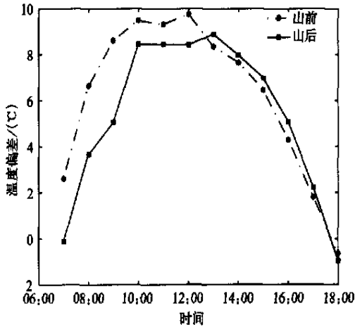
图7 山前山后的地面与参考层(10m)温差日变化
